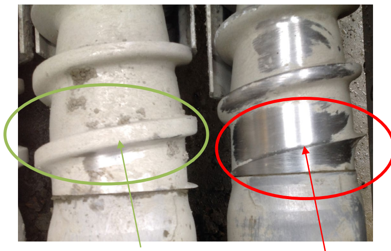
Медленный износ спирали Новая спираль Изнанная спираль, требующая замены
