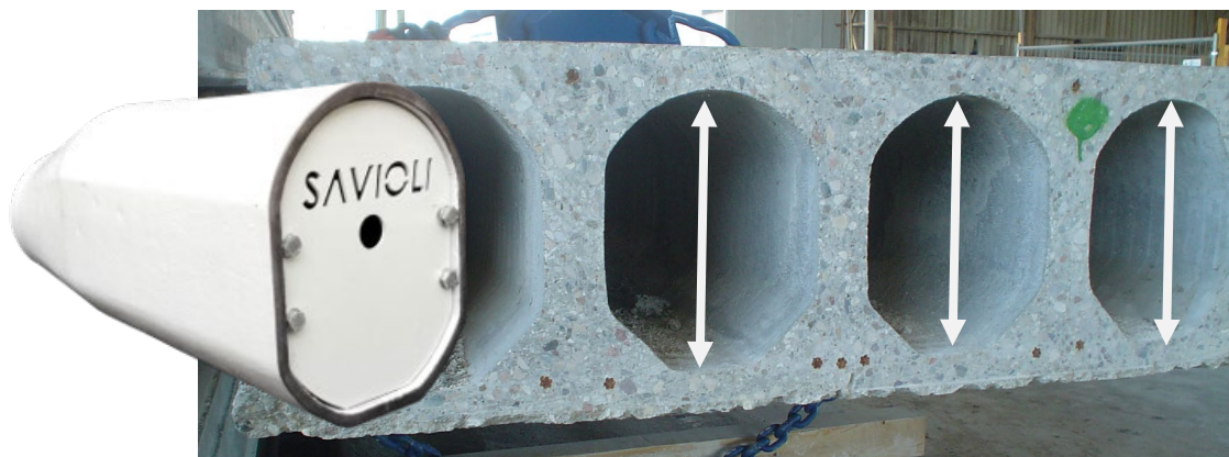
Отличная формовка отверстий в плите
